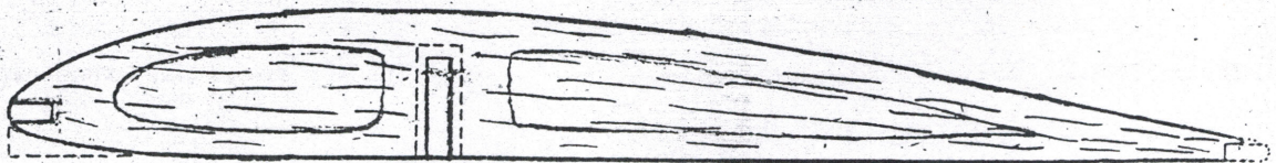
Žebro křídla ve skutečné velikosti. (Čárkované čáry platí pro dvě střední žebra.)
